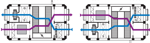
Configuration L sauf EVERKIT® 5000
