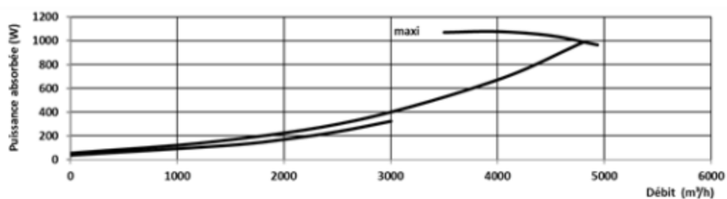
Figure 50 - ECOVOR® 5000 LOBBY (triphasé)
