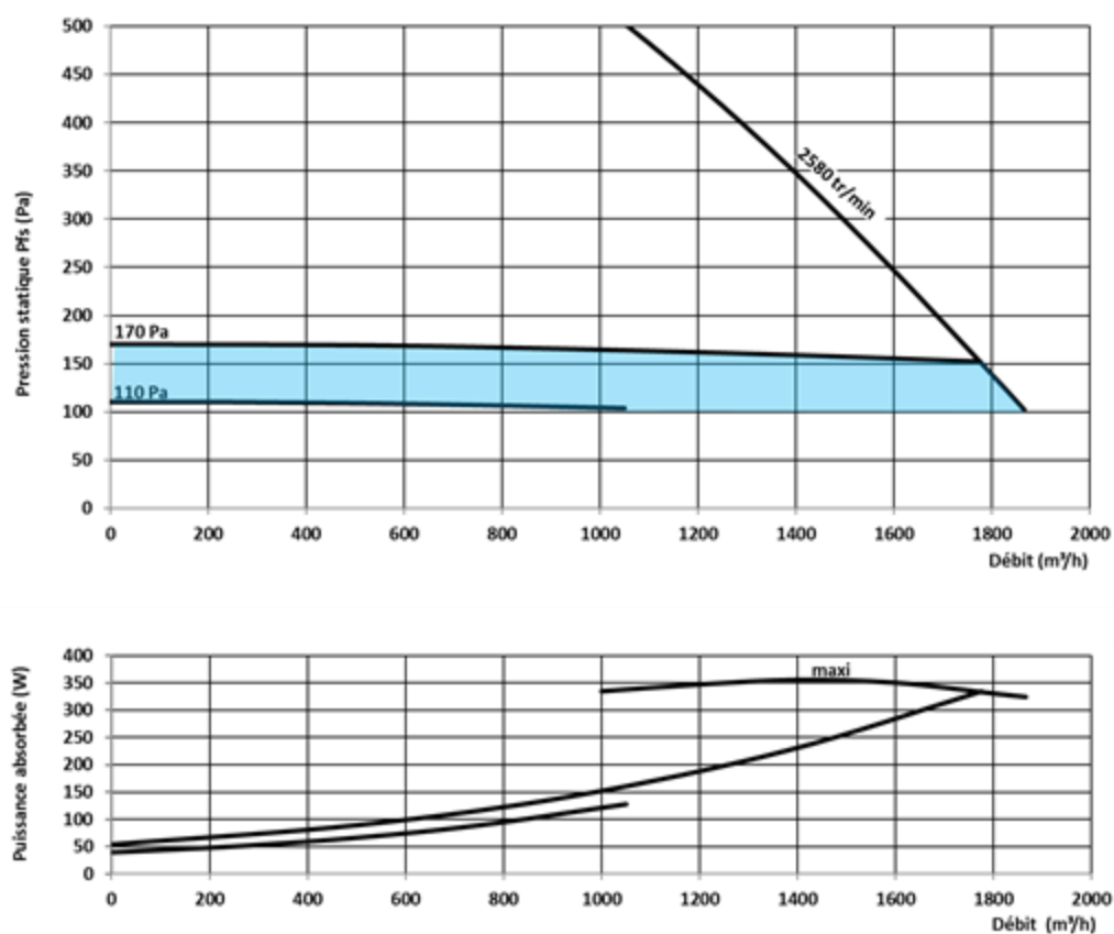
Figure 48 - ECOVOR® 1500 LOBBY (monophasé)
