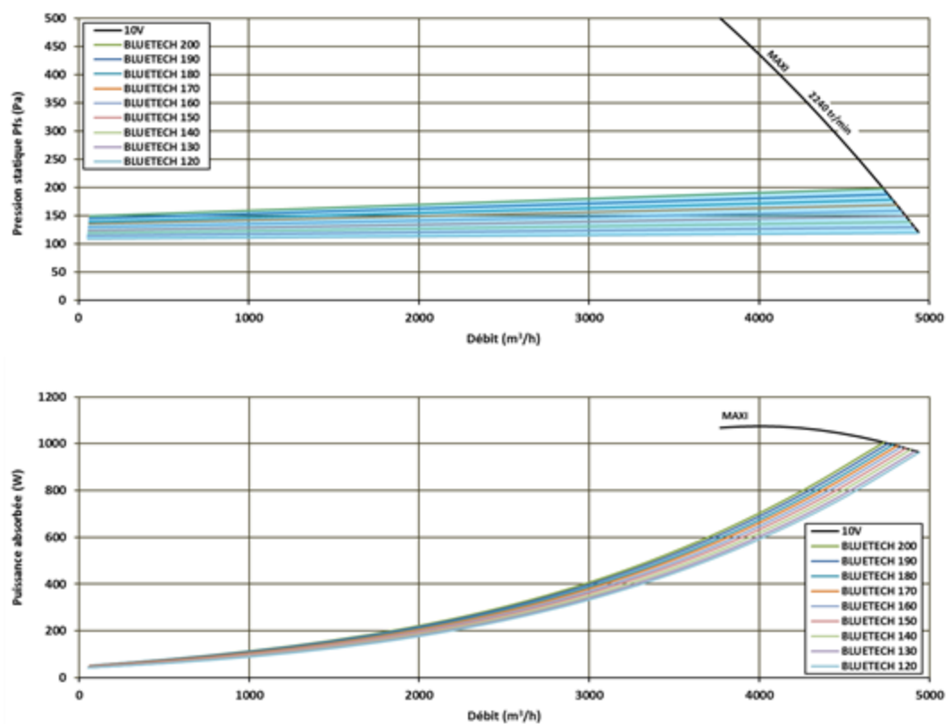
Figure 53 - ECOVOR® 5000 BLUETECH (triphasé)
