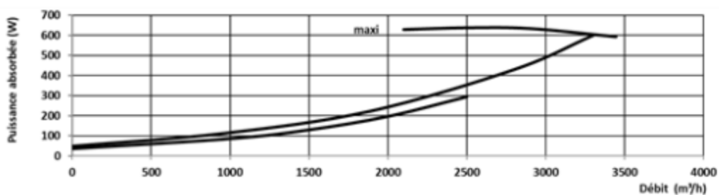
Figure 49 - ECOVOR® 3000 LOBBY (monophasé)
