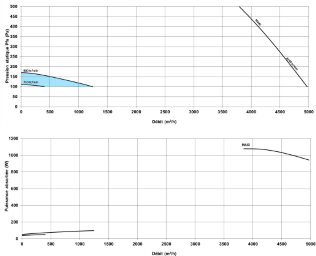
Figure 59 - ECOVOR® 5000 ECONIZER (triphasé)
