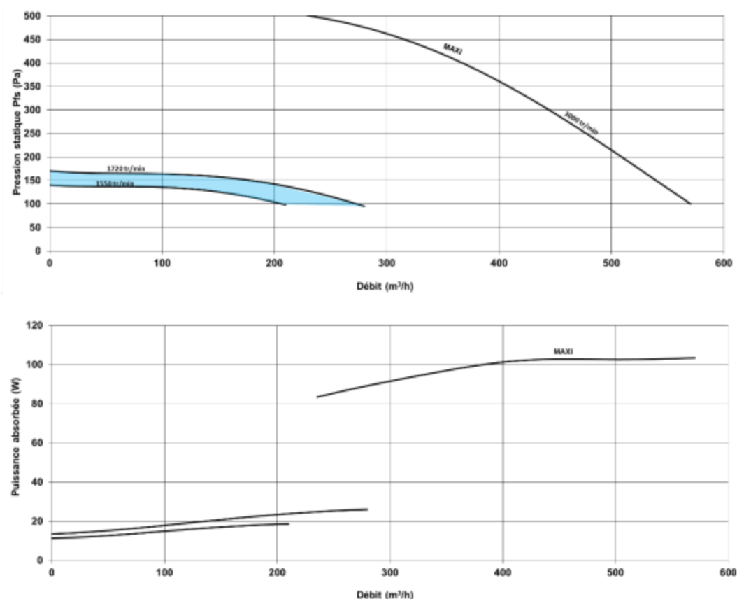
Figure 54 - ECOBLUE® 600 ECONIZER (OU ECONIZER 600)
