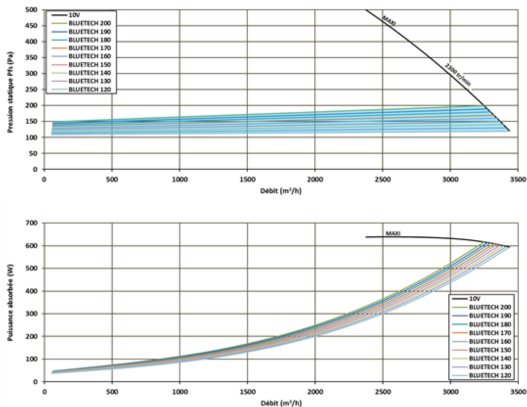
Figure 52 - ECOVOR® 3000 BLUETECH (monophasé)
