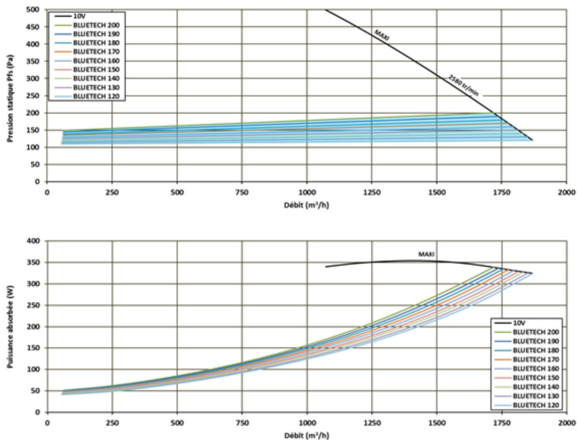
Figure 51 - ECOVOR® 1500 BLUETECH (monophasé)
