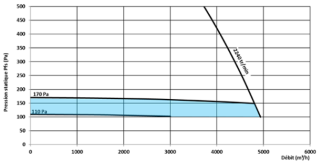
Figure 49 - ECOVOR® 3000 LOBBY (monophasé)
