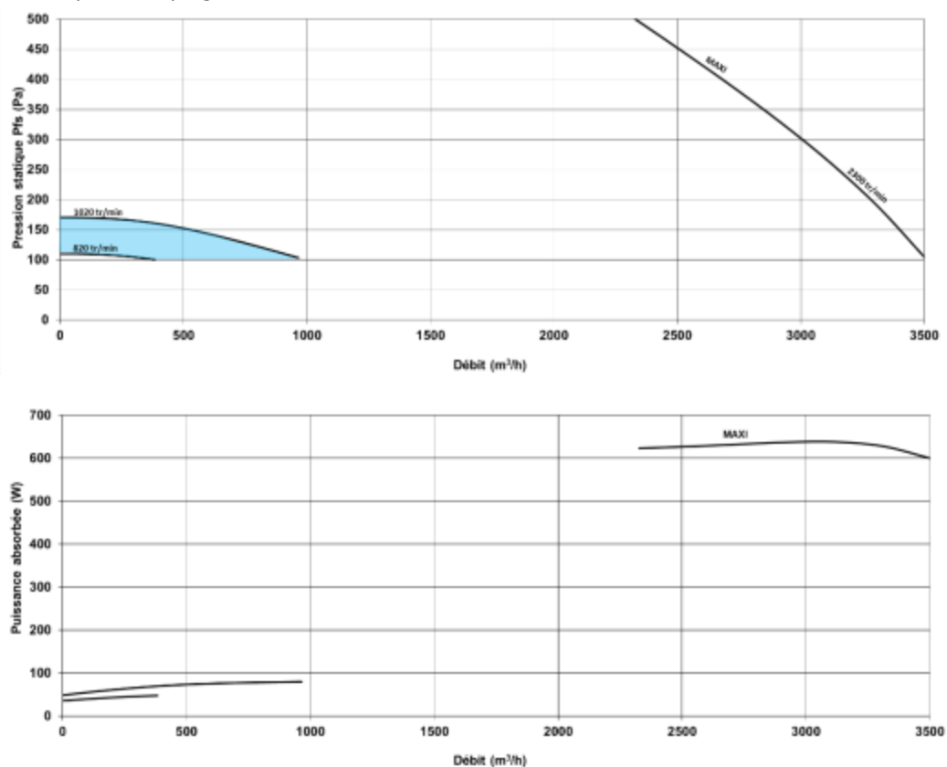
Figure 57 - ECOVOR® 3000 ECONIZER (monophasé)
