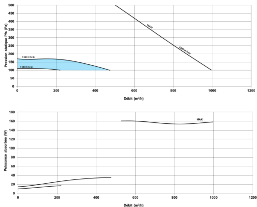
Figure 55 - ECOBLUE® 1000 ECONIZER (OU ECONIZER 1000)
